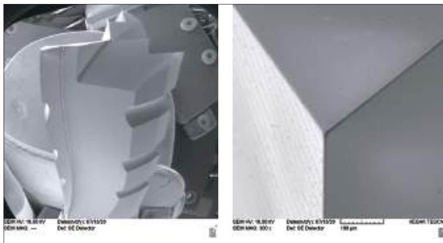
DLC 3 -beschichteter Schaftfräser unter dem Rasterelektronenmikroskop.
