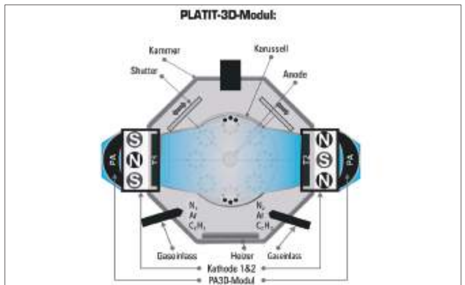
Die hochproduktive DCMS- und HiPIMS-Beschichtungsanlage PL711 von PLATIT.
